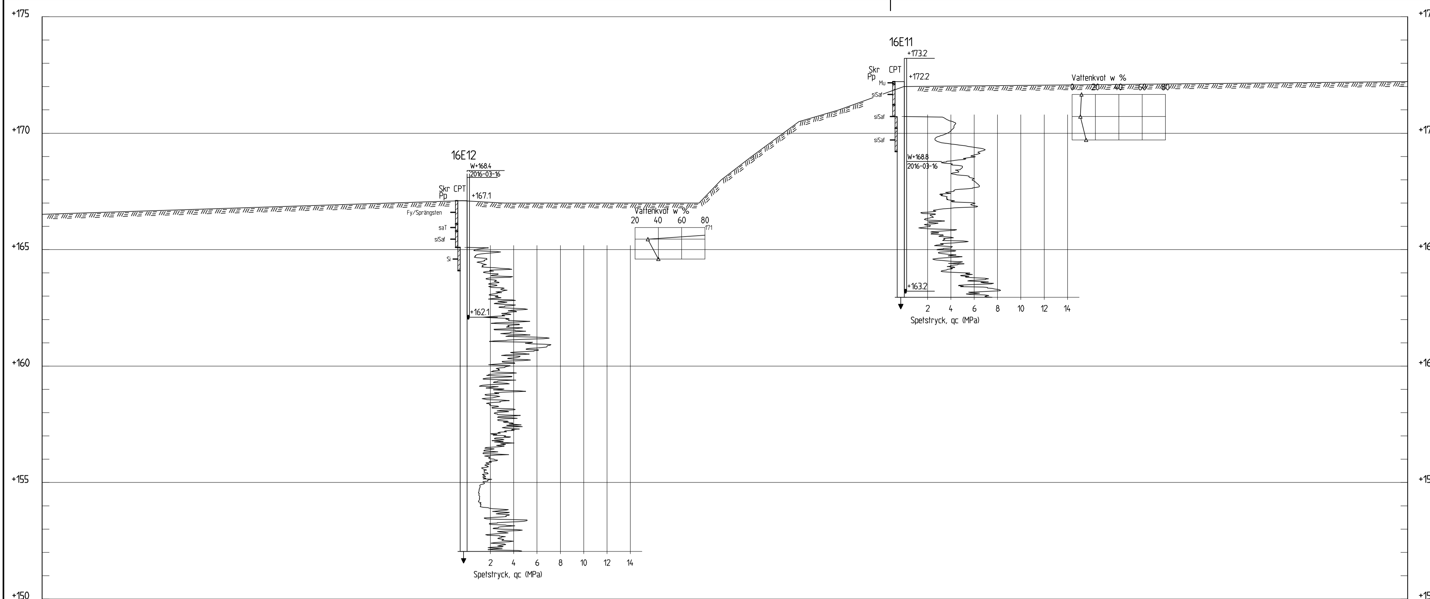
SEKTION A-A 1: 100
