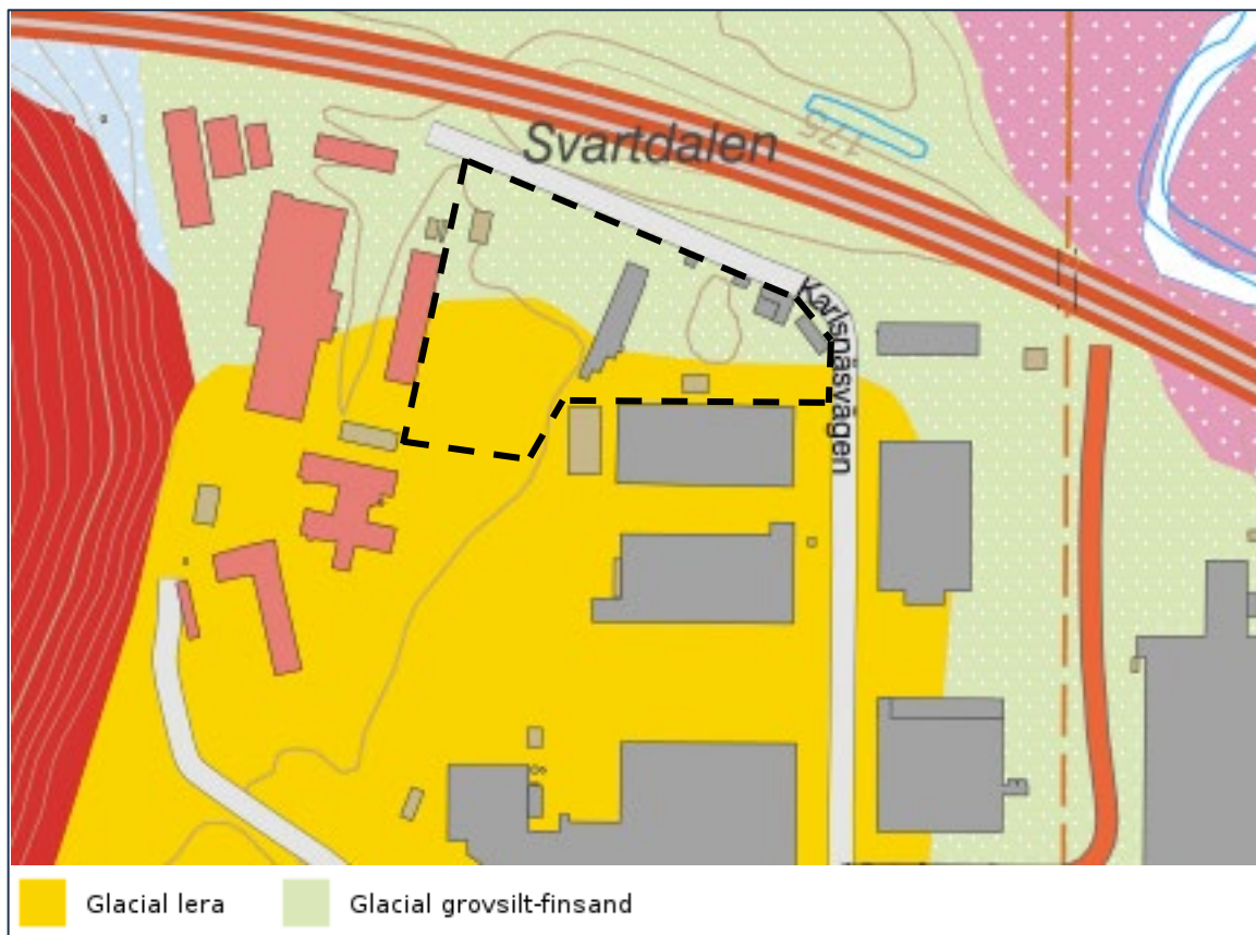
Figur 3: Urklipp från jordartskartan där undersökningsområdet är översiktligt markerat med svart streckad linje, Källa: ©SGU (Sveriges Geologiska Undersökning 2024).
