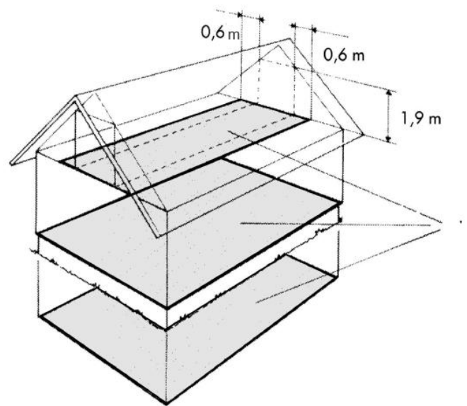
Bruttoarea (BTA)
